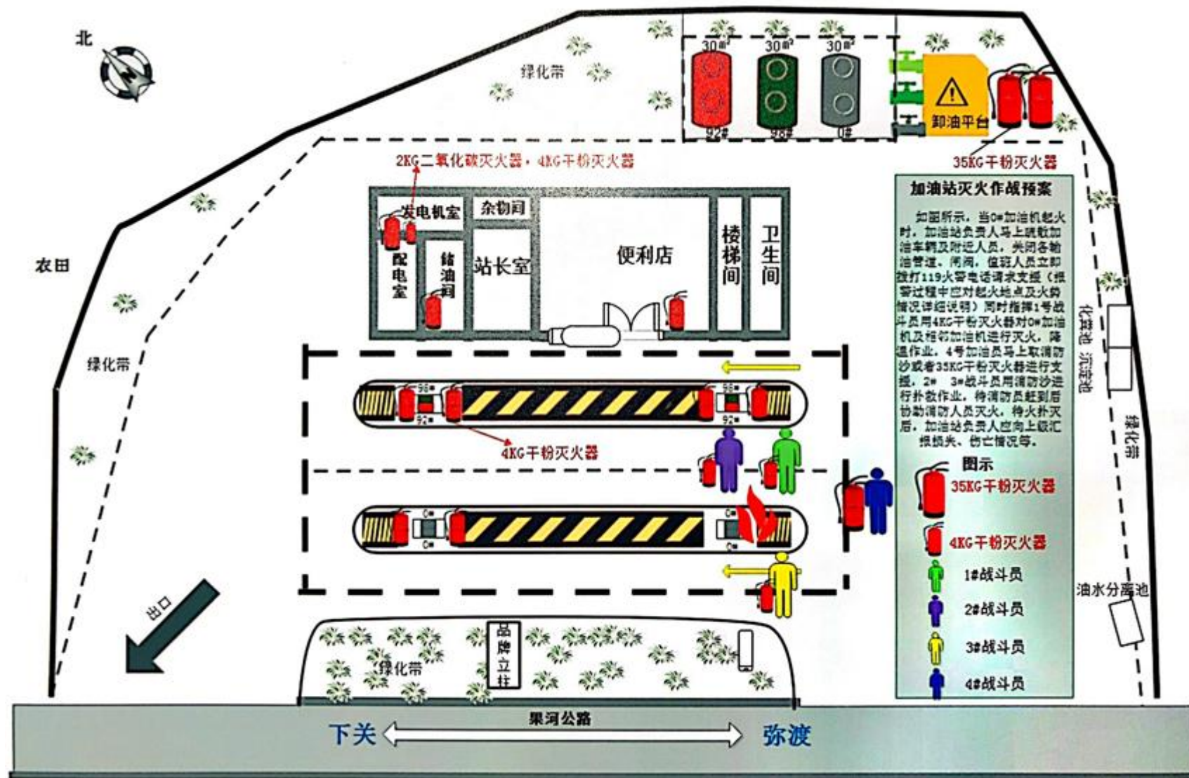
附图 5 加油站灭火作战图
