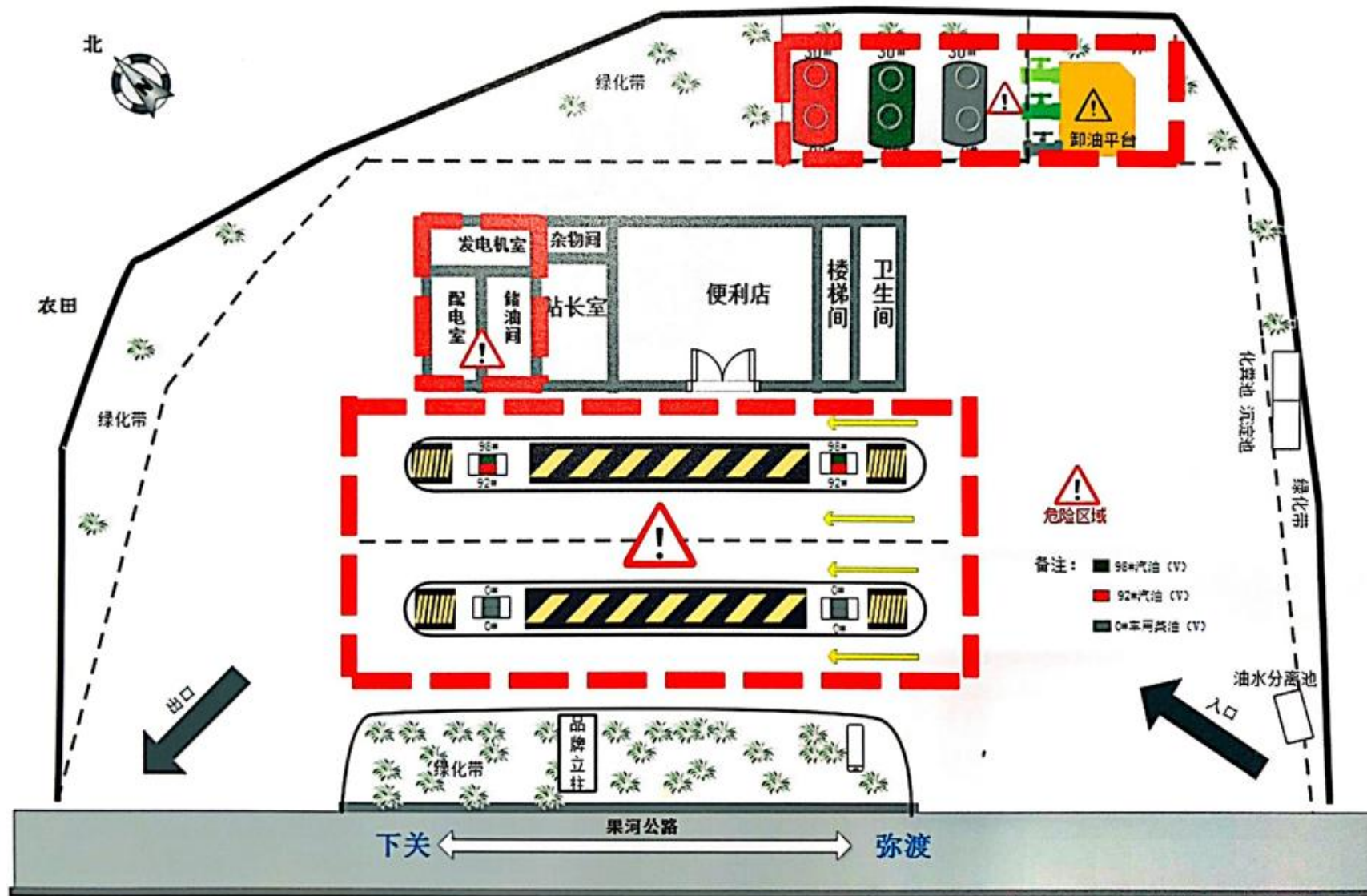
附图 4 加油站消防布置图
